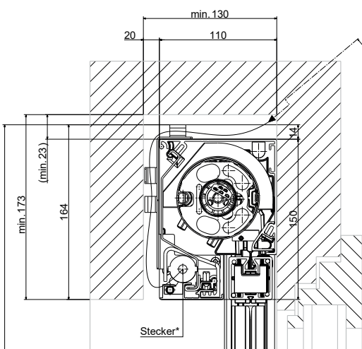
VS ZIP Pro S (110 mm) Dans le linteau creux avec coulisse standard
