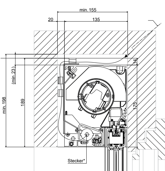
VS ZIP Pro L (135 mm) Dans le linteau creux avec coulisse standard
