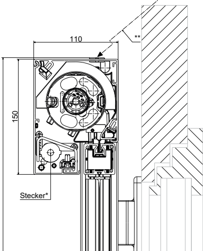
VS ZIP Pro S (110 mm) Caisson avec coulisse sur support de coulisse
