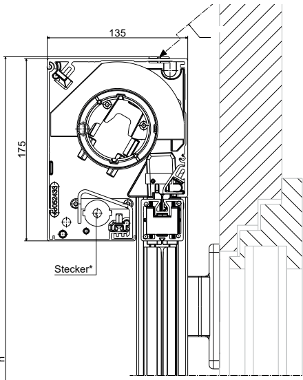
VS ZIP Pro L (135 mm) Caisson avec coulisse sur support de coulisse
