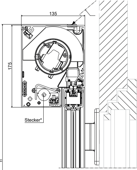
VS ZIP Pro L (135 mm) Avancorpo con guida su squadrette per guida
