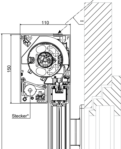
VS ZIP Pro S (110 mm) Avancorpo con guida su squadrette per guida
