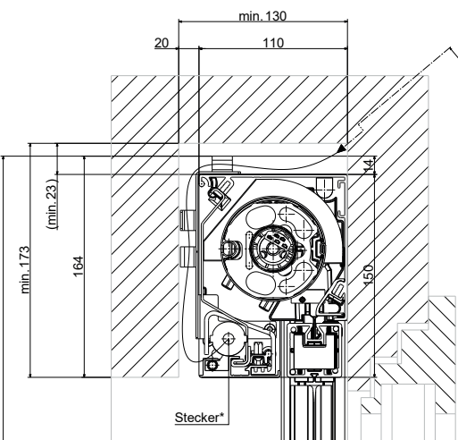
VS ZIP Pro S (110 mm) In architrave incavato con guida standard
