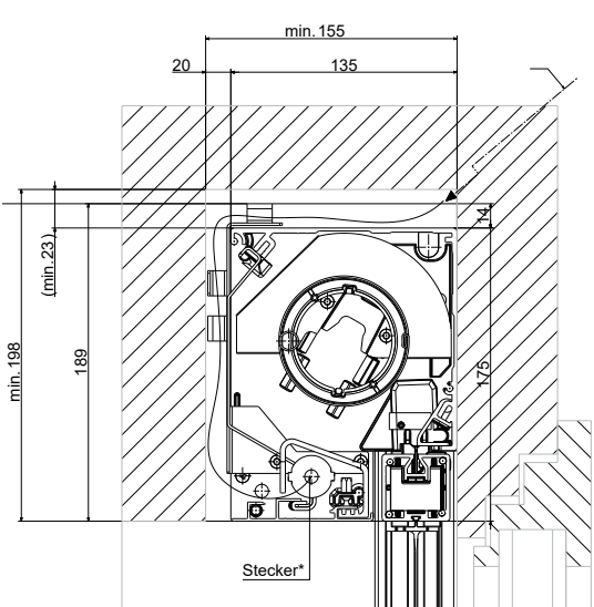
VS ZIP Pro L (135 mm) In architrave incavato con guida standard
