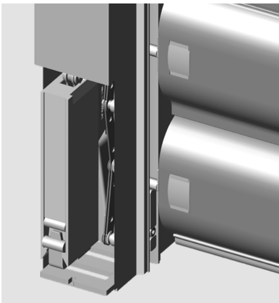
^ In der Laibung integrierte Führung für noch mehr Ästhetik (optional)
