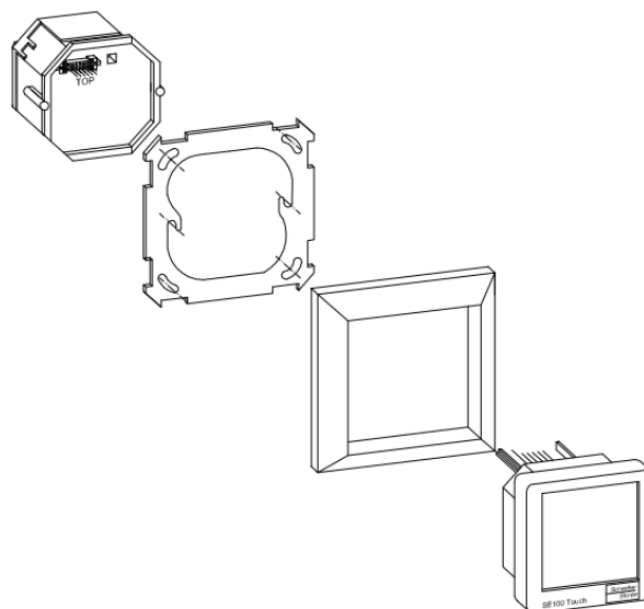
Abbildung 3: Aufbau Steuerzentrale SE 100 Touch
