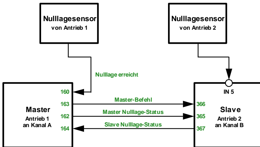
Abbildung 9: Master-Slave-Verriegelung Beispiel 3
