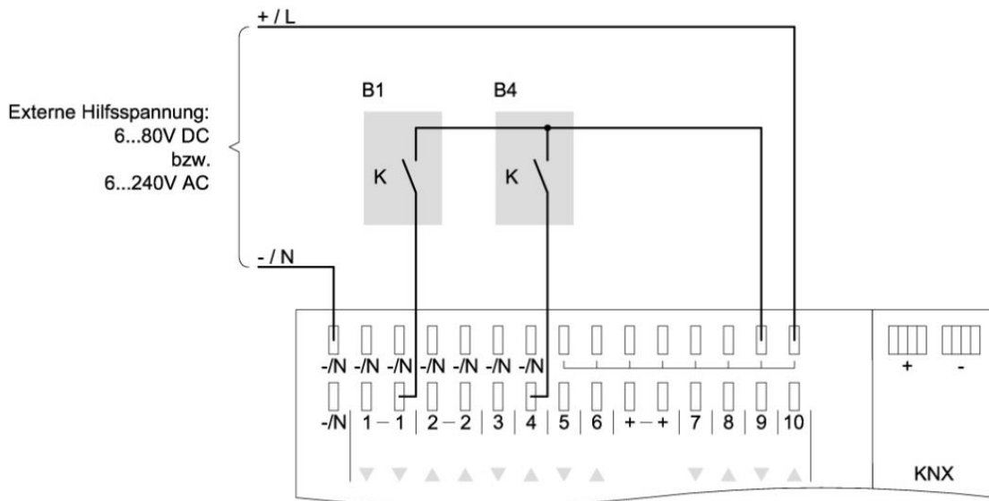
Abbildung 5: Nutzung einer externen Hilfsspannung für Binäreingänge
