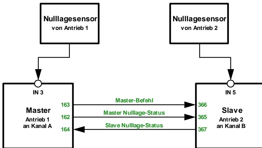
Abbildung 7: Master-Slave-Verriegelung Beispiel 1
