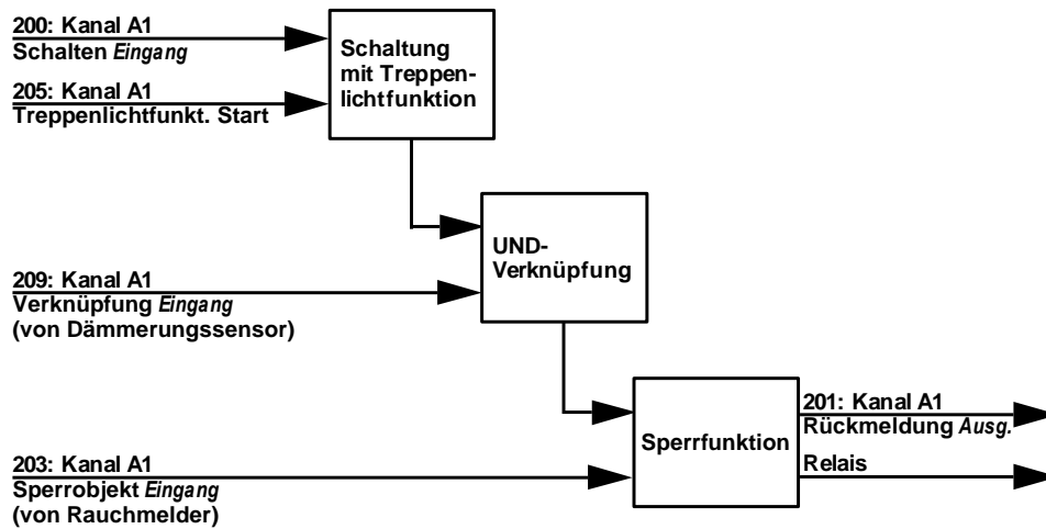
Abbildung 11: Beispiel Schaltausgang Verknüpfung – Zeitschalten – Sperre
