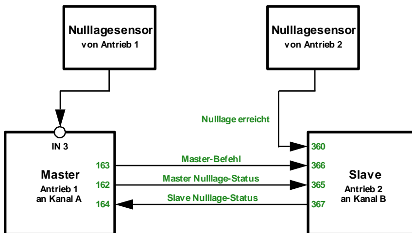
Abbildung 8: Master-Slave-Verriegelung Beispiel 2
