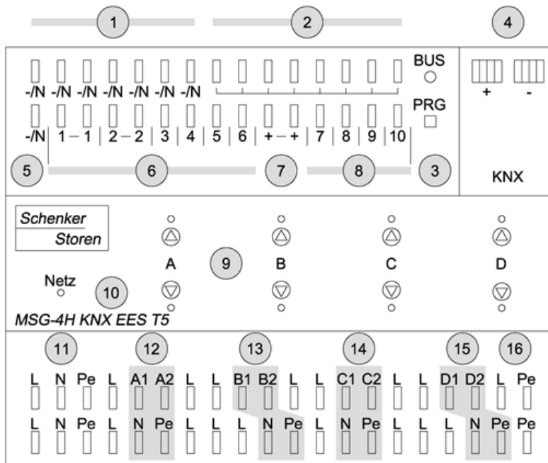
Abbildung 3: Aufbau MSG-4H KNX EES T5
