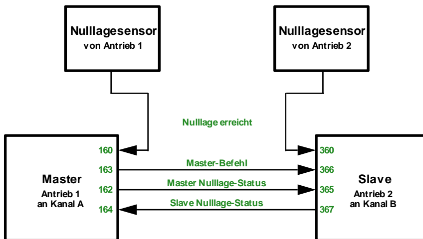
Abbildung 10: Master-Slave-Verriegelung Beispiel 4
