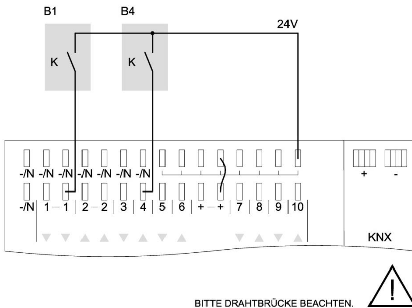
Abbildung 4: Nutzung der internen Hilfsspannung für Binäreingänge
