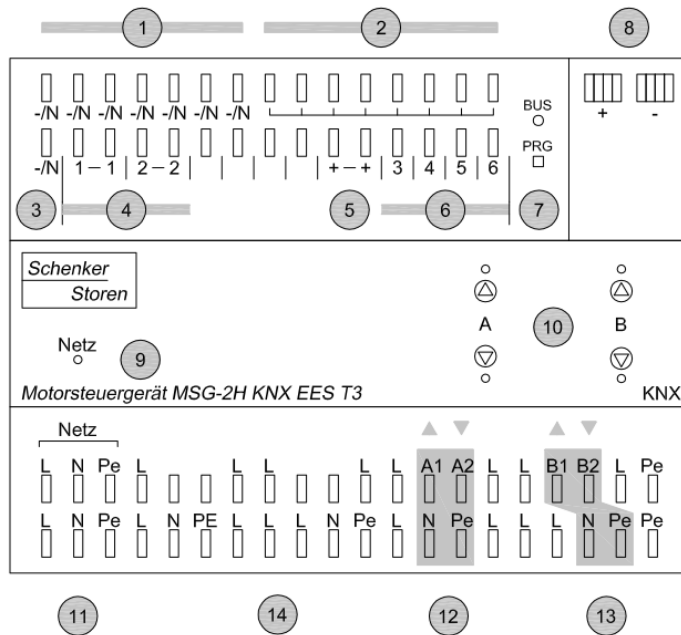
Abbildung 2: Aufbau MSG-2H KNX EES T3
