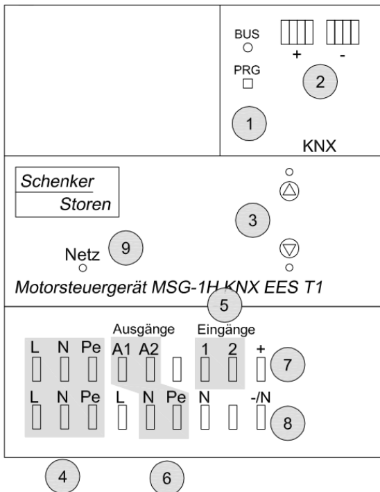
Abbildung 1: Aufbau MSG-1H KNX EES T1
